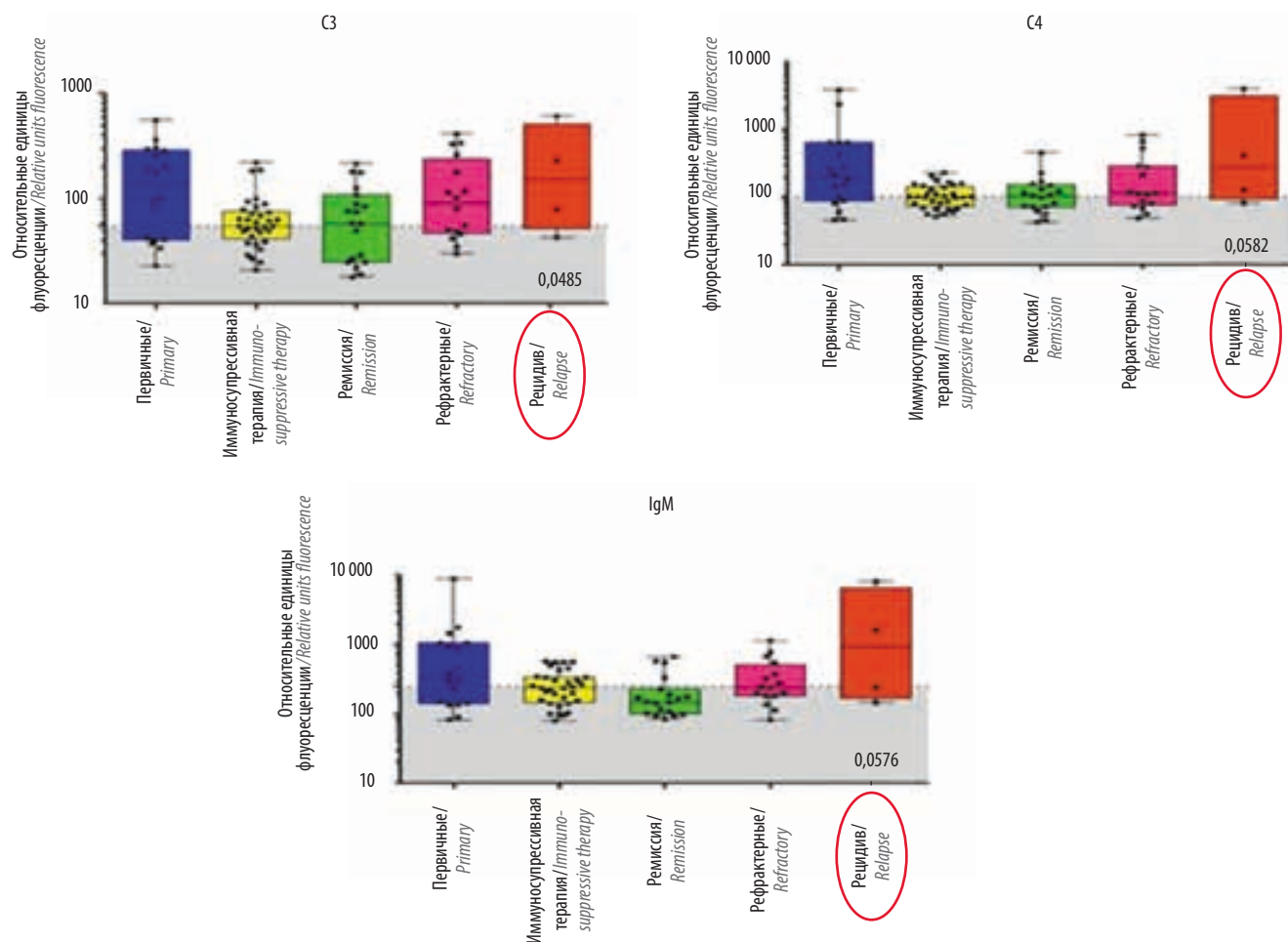
Рис. 6. Значения средней интенсивности флуоресценции тромбоцитассоциированных иммуноглобулинов и компонентов системы комплемента в зависимости от степени тяжести заболевания и клинического статуса
