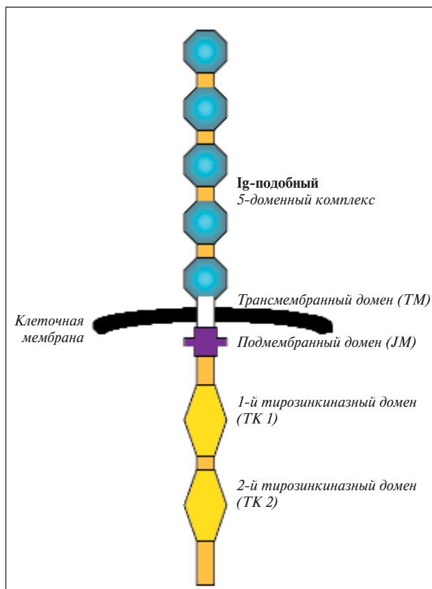
Рис. 1. Схема строения одиночной молекулы рецептора FLT3
