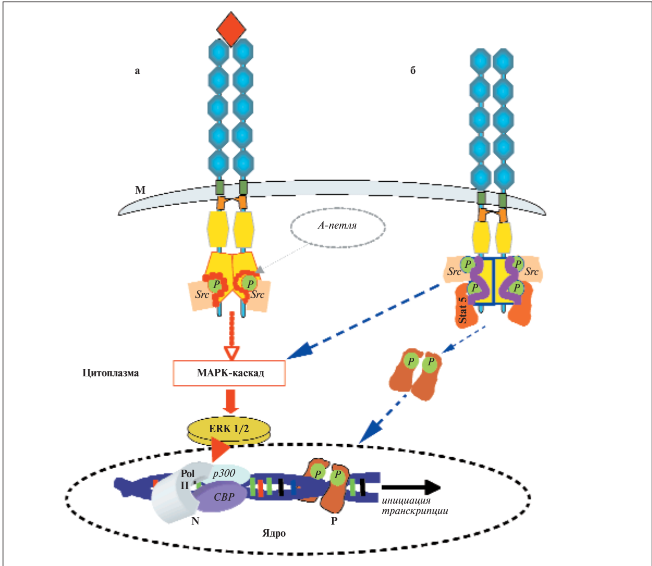
Рис. 2. Схематическое изображение активации FLT3
